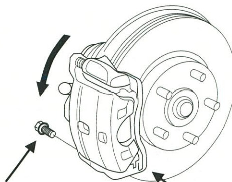
フランジ ボルト トルク 34N・m(3.5kgf・m)
