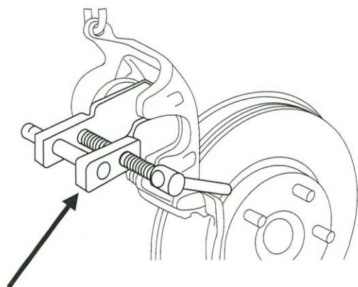
ブレーキ キャリパ レンチ
